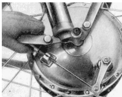
Bild 46. Vorderradbremse nachstellen
