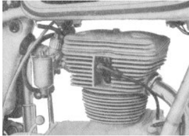
Bild 8. Zylinderkopf und Zylinder
