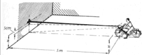
Bild 52. Einstellen des Scheinwerfers
