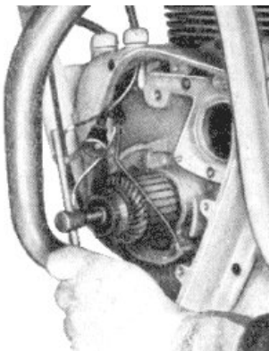
Bild 87. Lichtmaschinenanker abdrücken
