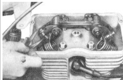
Bild 14. Kontrolle des Ventilspiels mittels Blattlehre
