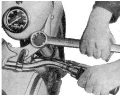
Bild 64. Lösen der Muttern zum Tragrohr
