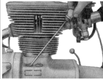
Bild 60. Ölstand im Motor prüfen
