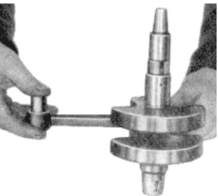
Bild 82. Der Kolbenbolzen darf in dieser Stellung nicht selbst durchsinken, er muß sich aber mit leichtem Fingerdruck durchdrücken lassen
