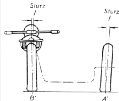
Bild 98. Einstellung des Seitenwagens (Sturz)
