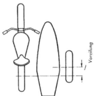
Bild 97. Einstellung des Seitenwagens (Voreilung)
