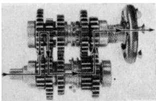
Bild 33. Räder in Schaltstellung 3. Gang
