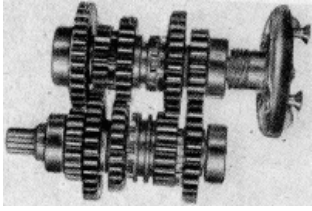
Bild 30. Räder in Leerlaufstellung
