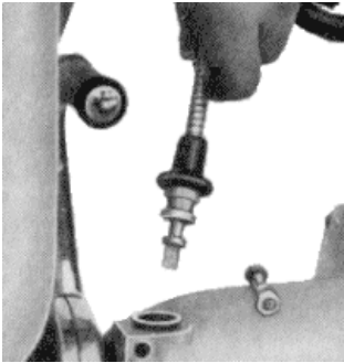
Bild 69. Ausbau der Tachometerantriebswelle
