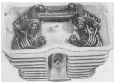
Bild 9. Blick in das offene Ventilgehäuse
