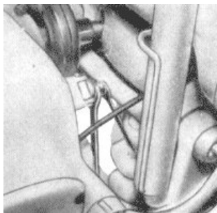
Bild 26. Einstellen der Druckschraube am Kupplungshebel
