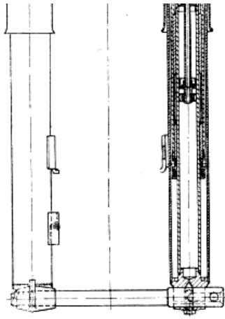
Bild 41. Schnittzeichnung Vordergabel
