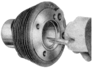
Bild 81. Kolbenringstoß prüfen
