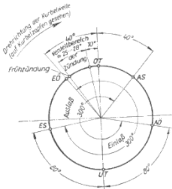
Bild 13. Steuerwinkeldiagramm
