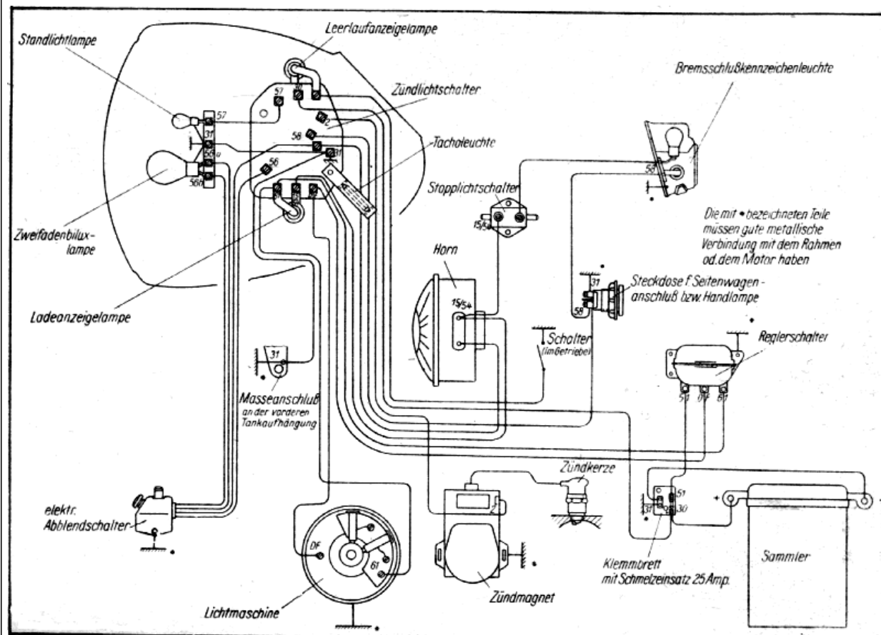
Bild 49. Schaltplan
