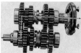
Bild 34. Räder in Schaltstellung 4. Gang
