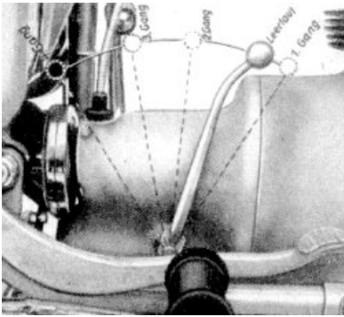
Bild 57. Handschalthebel
