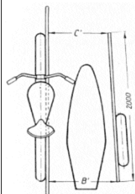
Bild 99. Einstellung des Seitenwagens (Vorspur)
