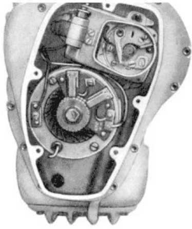
Bild 47. Elektrikgehäuse mit Lichtmaschine und Magnetzündler
