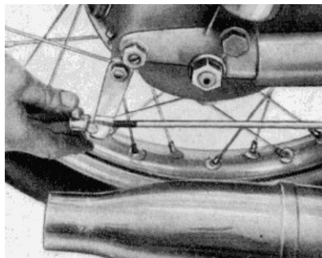
Bild 45. Hinterradbremse nachstellen
