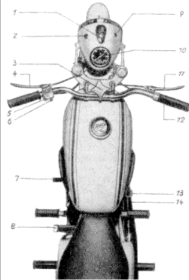
Bild 54. Anordnung der Bedienungselemente
