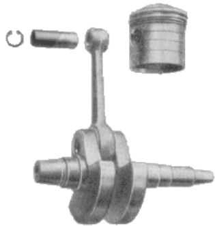
Bild 5. Kurbeltrieb
