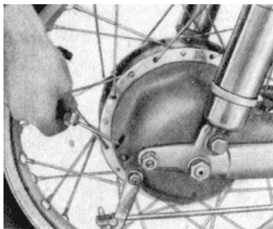
Bild 62. Ölstand im Hinterradantrieb prüfen
