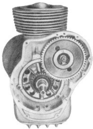
Bild 12. Antrieb der Steuerwelle
