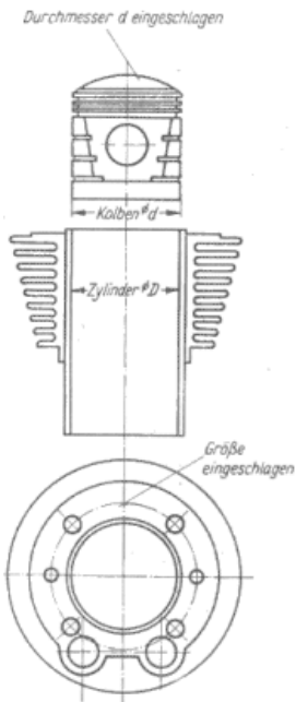
Bild 7. Aufstellung des Kolbeneinbauspiels
