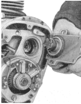
Bild 86. Magnetzünder ausbauen
