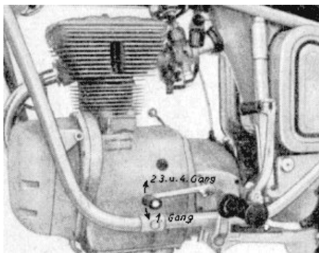
Bild 56. Fußschalthebel
