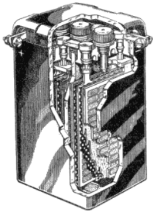
Bild 50. Bleibatterie 6 V, 8 Ah, (K 20)
