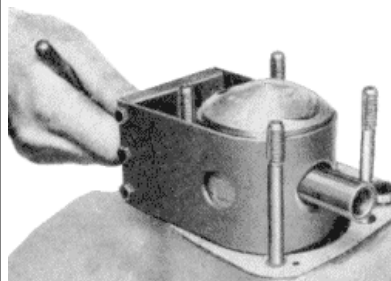
Bild 79. Kolbenbolzen ausdrücken
