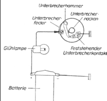
Bild 75. Schaltschema zur Einstellung der Zündung mittels Prüflampe
