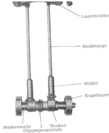
Bild 11. Ventilsteuerung der AWO 425 S
