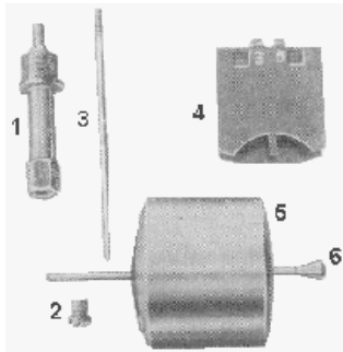
Bild 20. Die wichtigsten Teile des Vergasers
