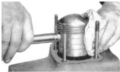
Bild 83. Einbau des Kolbenbolzens mittels Hilfsdornes
