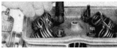
Bild 63. Zuganker für Zylinderkopf nachziehen
