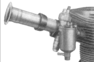
Bild 17. Vergaser mit Ansaugrohr und Lufttrichter
