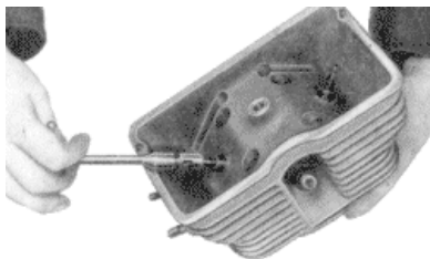
Bild 78. Ventile einschleifen
