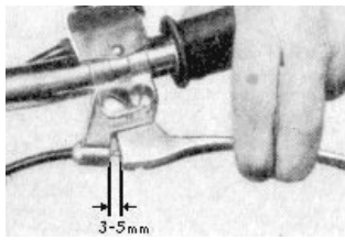
Bild 55. Erforderliches Spiel am Kupplungshebel
