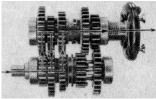
Bild 32. Räder in Schaltstellung 2. Gang
