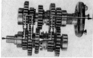
Bild 31. Räder in Schaltstellung 1. Gang
