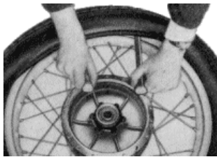
Bild 95. Reifen abnehmen
