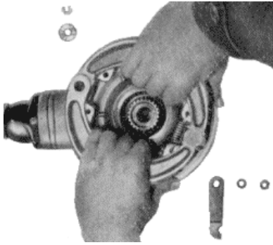
Bild 94. Bremsbacken abnehmen
