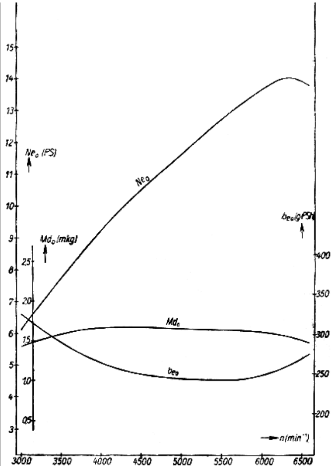
Bild 1. Motorkennlinien
