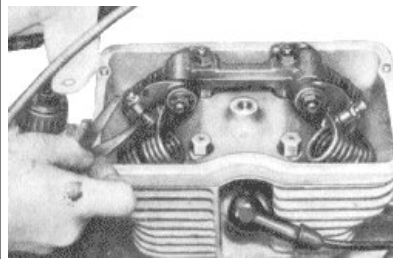
Bild 14. Kontrolle des Ventilspiels mittels Blattlehre
