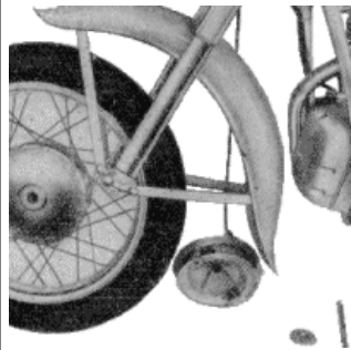
Bild 90. Vorderrad ausbauen
