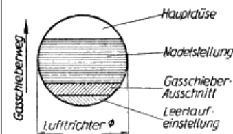
Bild 21. Wirkungsbereiche der verschiedenen Einstellfaktoren beim Vergaser
