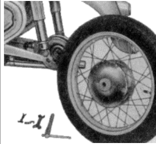
Bild 91. Hinterrad ausbauen
