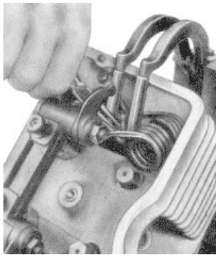
Bild 77. Ventile ausbauen
