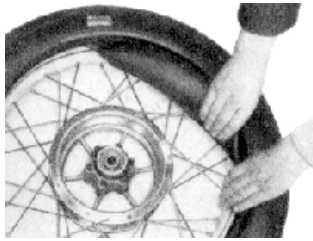
Bild 96. Schlauch einlegen
