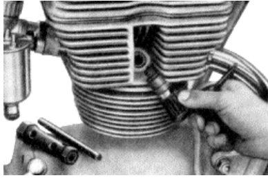
Bild 71. Zündkerze prüfen
