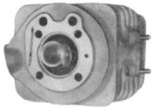
Bild 10. Verbrennungsraum mit geöffnetem Einlaßventil
