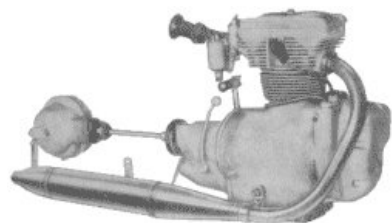
Bild 2. Antriebsblock der AWO 425 S
