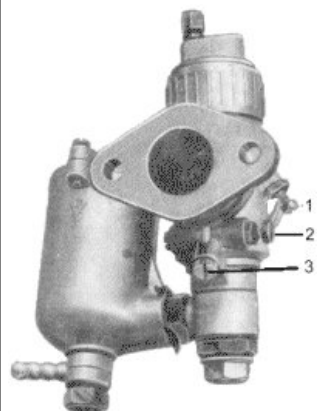
Bild 18 und 19. Zwei Vergaseransichten Gasschieberanschlagschraube (1), LeerlaufLuftschrabe (2),
